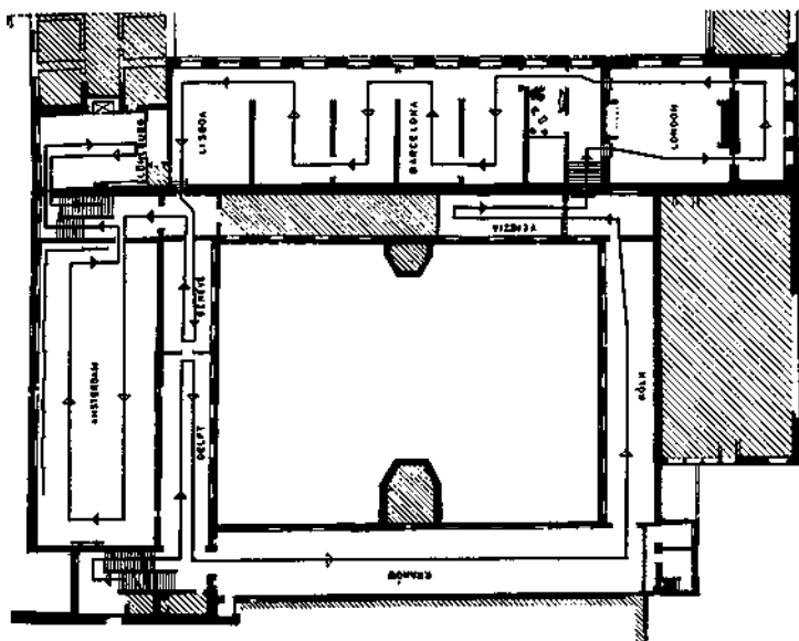
1 e VERDIEPING
